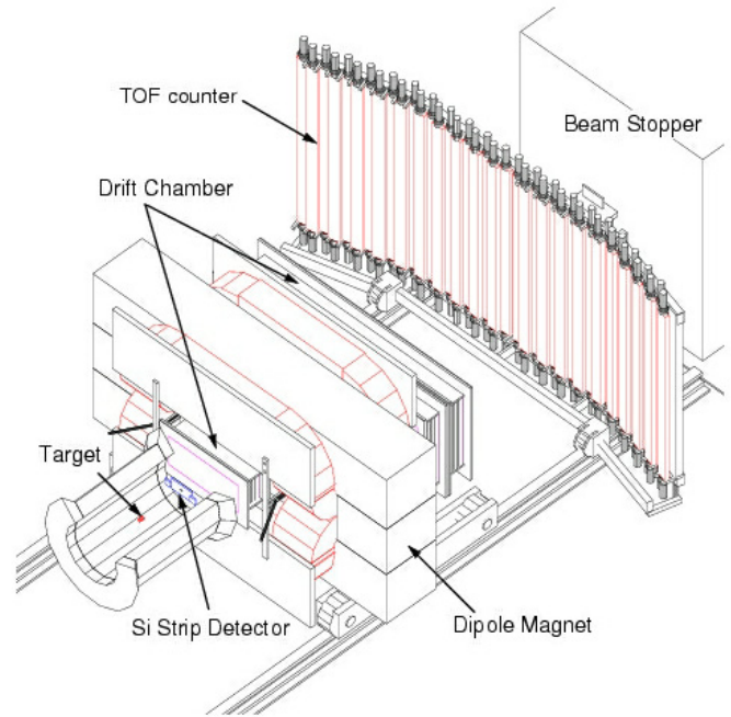
Fig. 2. The LEPS spectrometer
